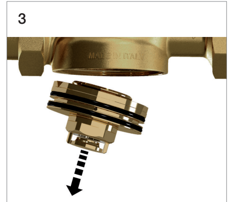
3 Rimuovere manualmente la cartuccia utilizzando guanti da lavoro. Sostituire con cartuccia 093D.
