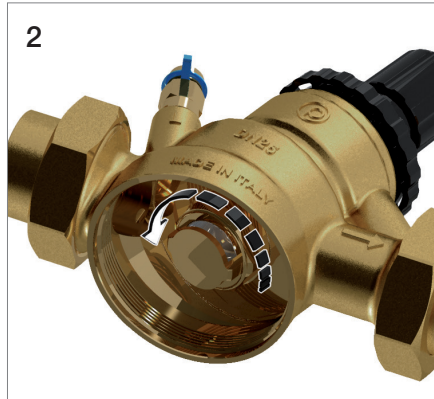
2 Svitare la cartuccia con una chiave esagonale
